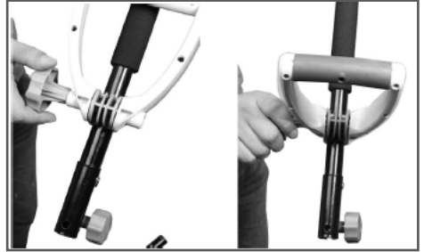
Рис. 5 Установка рабочей рукоятки
