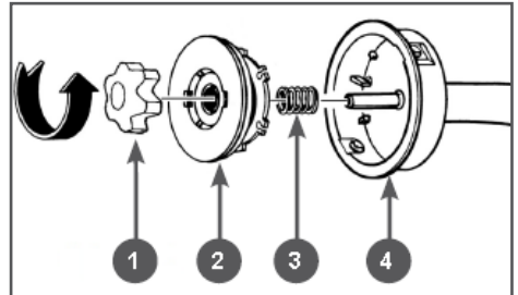
Рис. 10 Снятие триммерной головки
