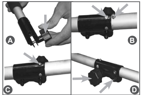
Рис. 6 Установка нижней штанги
