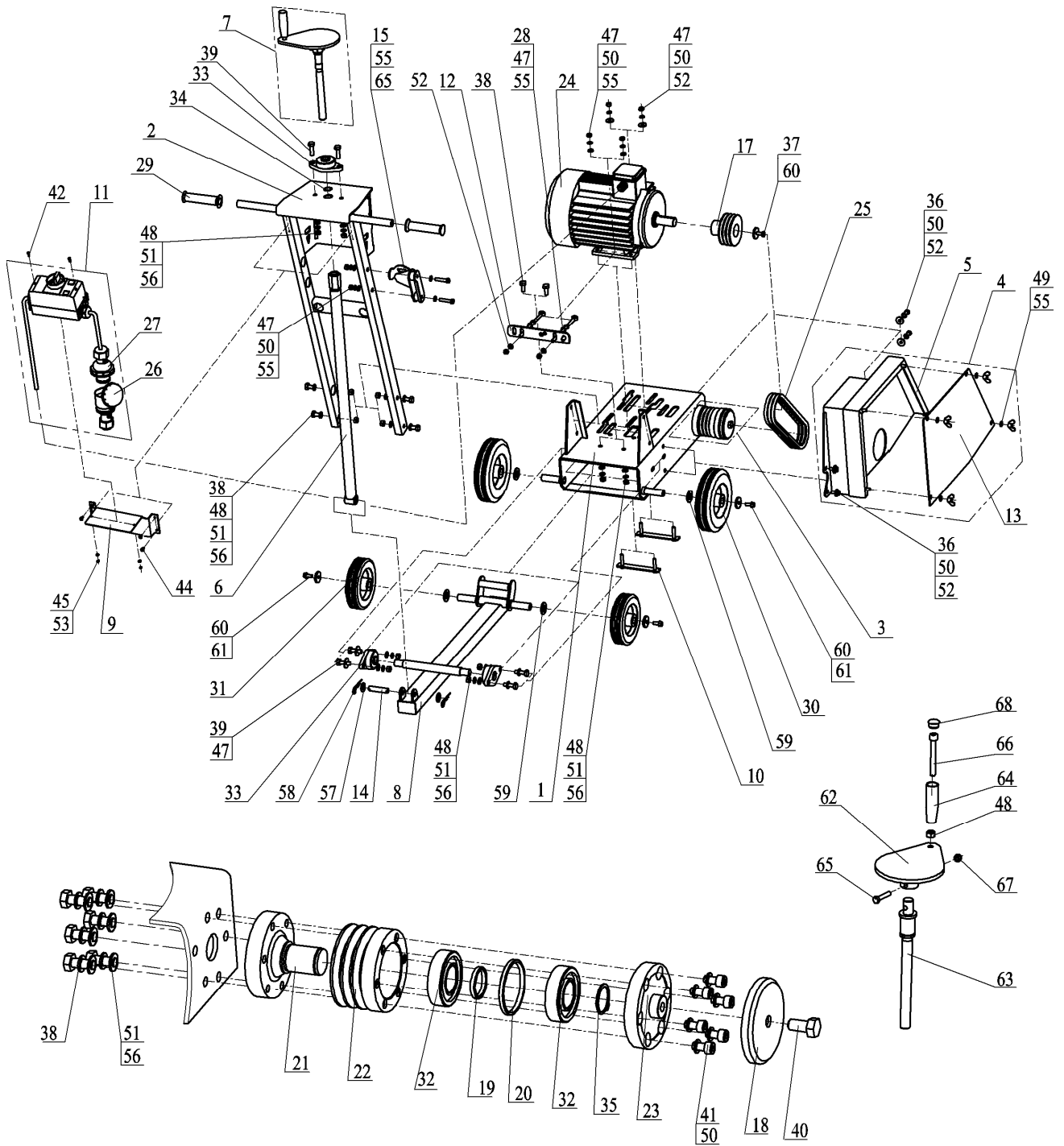
Рисунок 13 – Компонировка резчиков
